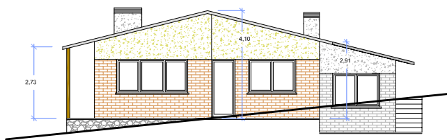
FAÇANA SUD
