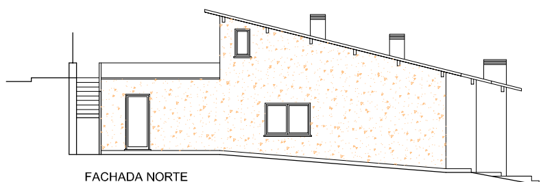
FACHADA NORTE
